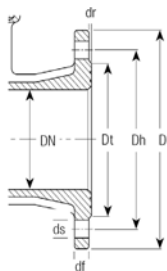
DN D Flensmaat mm Dt mm Dh Steekcirkel mm df Flensdikte mm dr mm ds Flensgat mm Aantal boutgaten Boutmaat PN10 PN16 PN10 PN16 PN10 PN16 PN10 PN16 PN10 PN16 PN10 PN16 PN10 PN16 40 150 83 110 16 3 19 4 M16 50 165 102 125 16 3 19 4 M16 65 185 122 145 16 3 19 4 M16 80 200 138 160 16 3 19 8 M16 100 220 158 180 16 3 19 8 M16 125 250 188 210 16 3 19 8 M16 150 285 212 240 16 3 23 8 M20 200 340 268 295 295 17 3 23 23 8 12 M20 250 400 320 350 355 19 3 23 28 12 12 M20 M24 300 455 370 400 410 21 4 23 28 12 12 M20 M24 350 520 430 460 470 23 4 23 28 16 16 M20 M24 400 580 482 515 525 28 4 28 31 16 16 M24 M27 450 640 530 548 565 585 28 4 28 31 20 20 M24 M27 500 715 582 609 620 650 28 4 28 34 20 20 M24 M30 600 840 682 720 725 770 29 5 31 37 20 20 M27 M33 700 895 910 800 795 840 840 28 35 5 31 37 24 22 M27 M33 800 1015 1025 905 900 950 950 30 38 5 34 41 24 24 M30 M36 900 1115 1125 1005 1000 1050 1050 33 42 5 34 41 28 28 M30 M36 1000 1230 1255 1110 1115 1160 1170 35 45 5 37 44 28 28 M33 M39 1200 1455 1485 1330 1330 1380 1390 40 52 5 41 50 32 32 M36 M45
